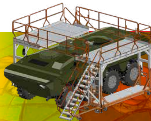
EM702 Estructura a Medida Estrutura à medida
