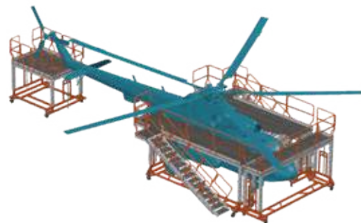
EM502 Escaleras Especiales Escadas especiais
