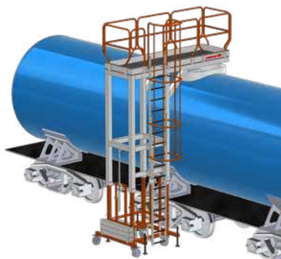
EM209 Estructura a Medida Estrutura à medida
