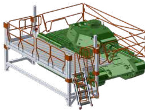
EM703 Plataforma a Medida Plataformas à medida
